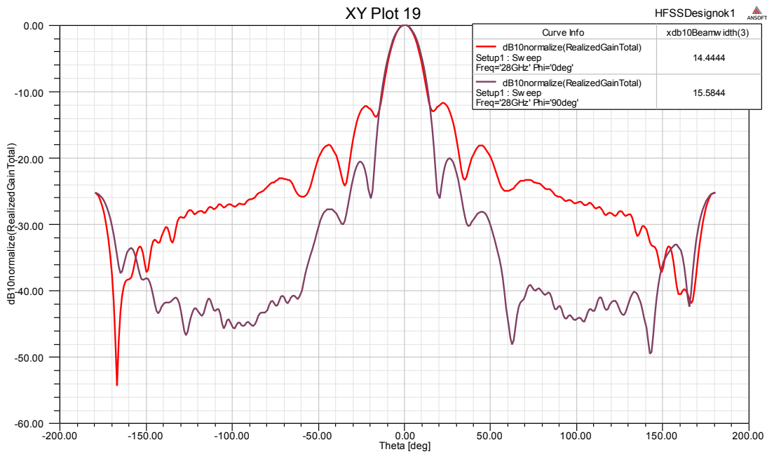
Gain@28GHz
